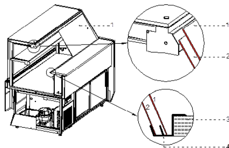
Rys.4 Montaż/demontaż przysłonek nocnych
