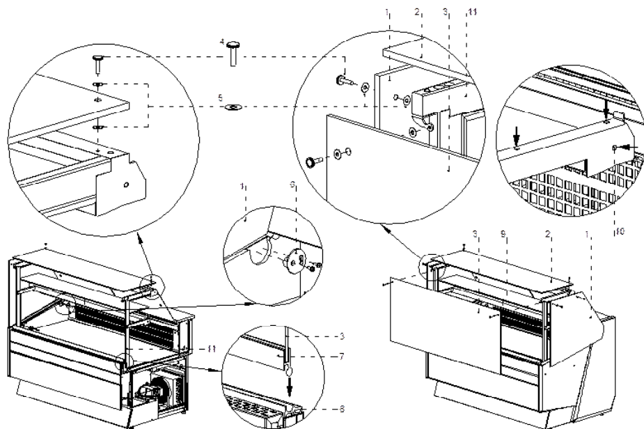
Rys.3 Mocowanie elementów szklanych
